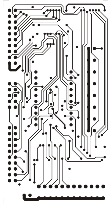
Leiterbild Lötseite
