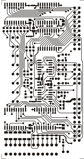
Leiterbild Bauteilseite
